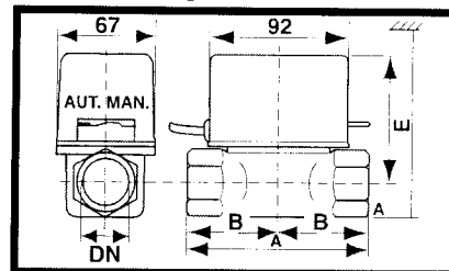
С внутренней резьбой
