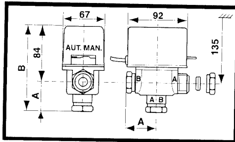
Ввод для Cu-трубок - EB
