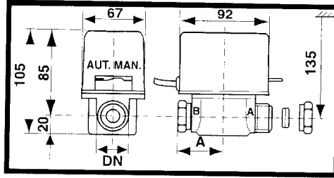
Ввод для Cu-трубок - EB
